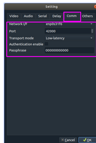
図 3-30 Comm タブ
