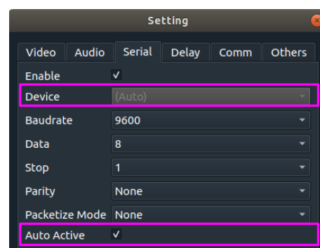
図 3-27 Auto Active
