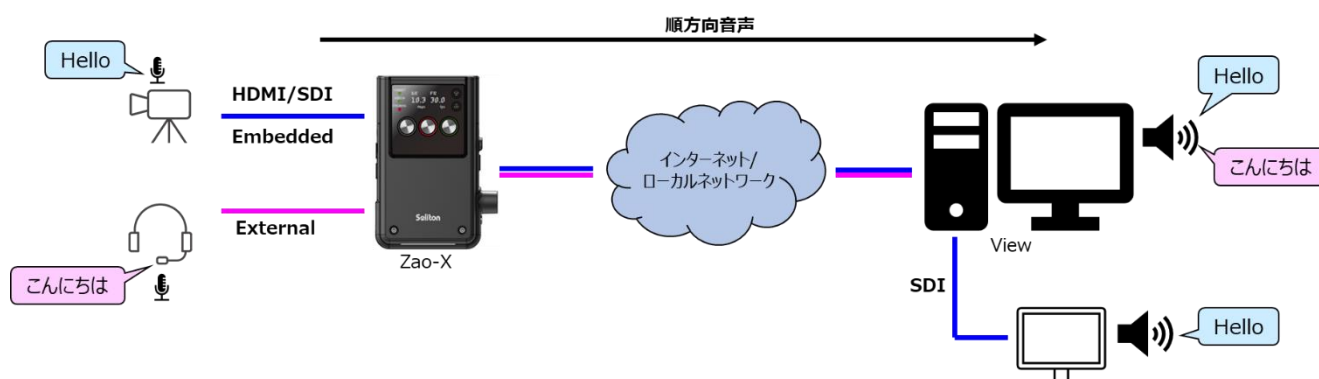
図 3-40 順方向音声
