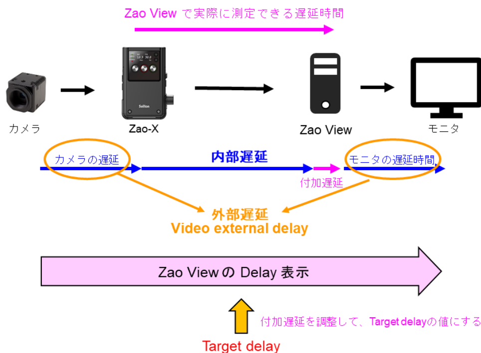
図 3-37 Delay 表示
