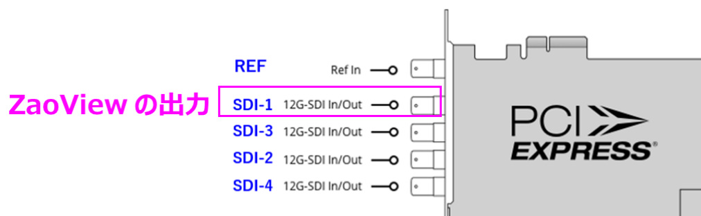
図 3-32 DeckLink 8K Pro の SDI 外部モニタとの接続ポート
