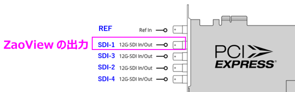
図 3-32 DeckLink 8K Pro の SDI 外部モニタとの接続ポート
