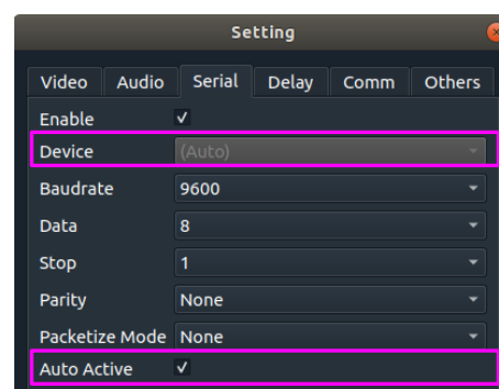
図 3-29 Auto Active
