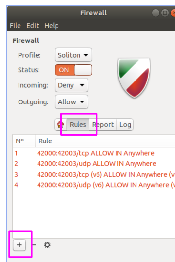
図 3-48 ファイアウォールの設定 1
