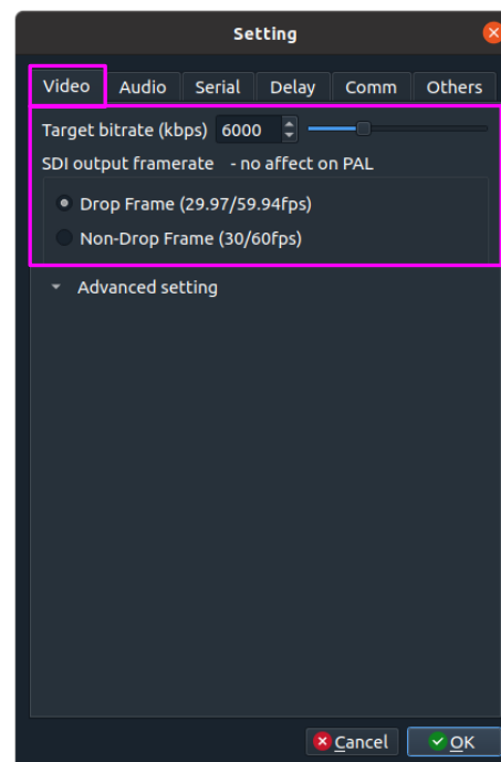
図 3-26 Video タブ
