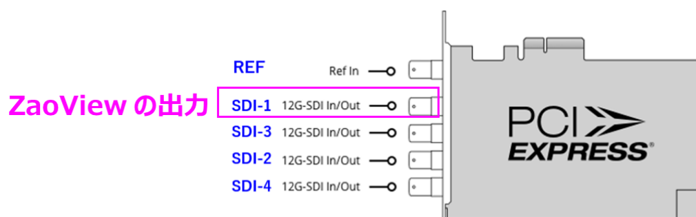
図 3-34 DeckLink 8K Pro の SDI 外部モニタとの接続ポート
