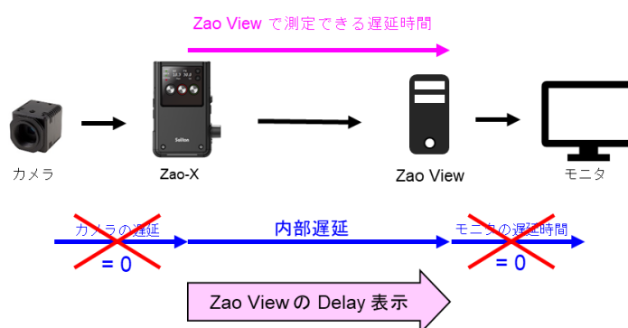
図 3-40 Video external delay 未設定
