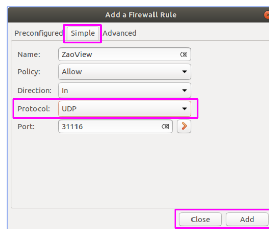
図 3-49 ファイアウォールの設定 2
