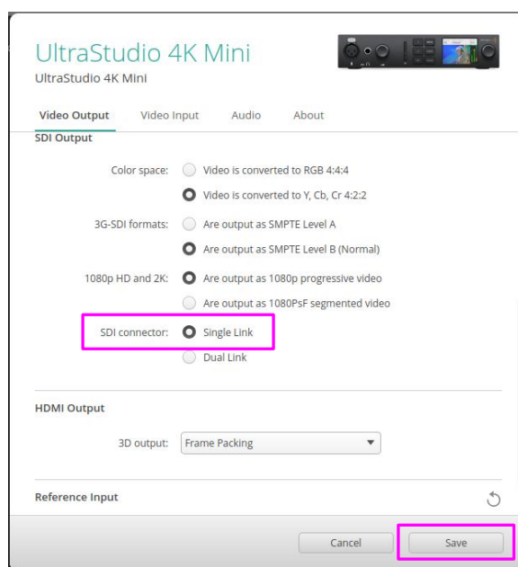
図 3-38 UltraStudio 4K Mini の設定画面
