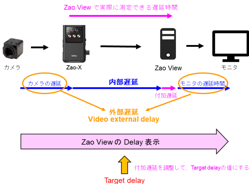
図 3-39 Delay 表示
