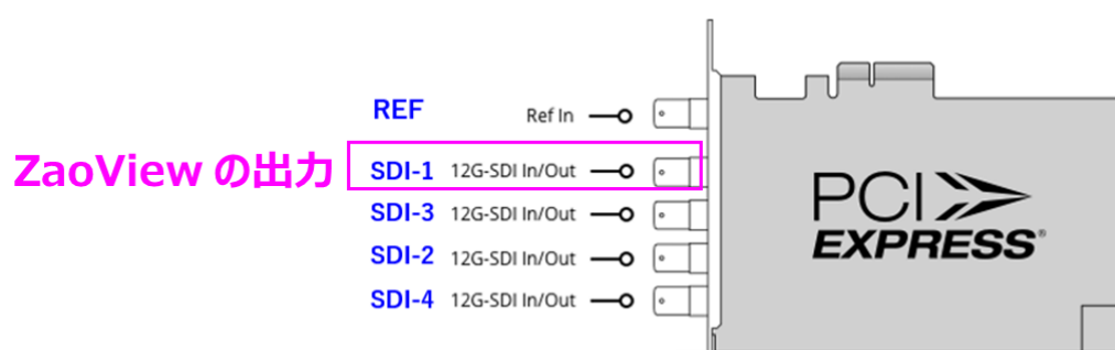
図 3-34 DeckLink 8K Pro の SDI 外部モニターとの接続ポート
